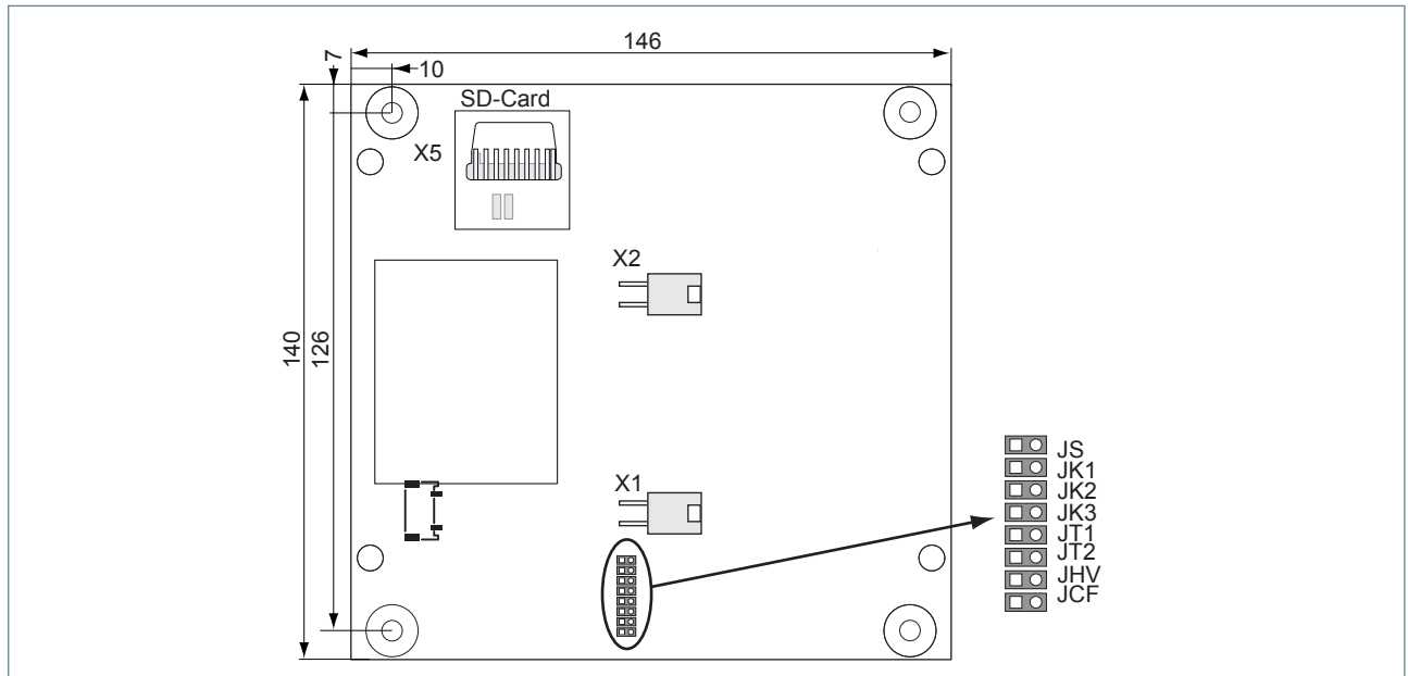
Abb. 2.1: Platinenzeichnung EAZ-TFT
